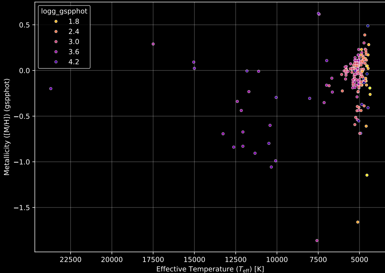
APOGEE DR17 Field: [154-04] Stellar Population Parameters (n= 205)
